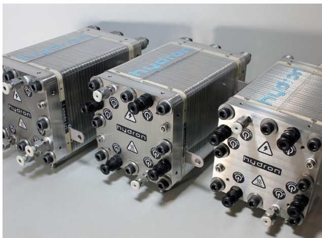
PEM-stacks
